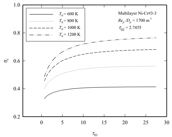
รูปที่ 1 ความสัมพันธ์ของประสิทธิภาพการแปลงรังสีความร้อนกับความหนาเชิงแสงของชั้นวัสดุพอรุน
