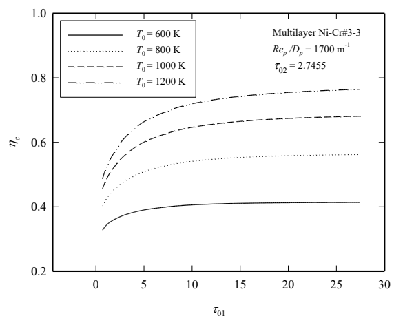
รูปที่ 1 ความสัมพันธ์ของประสิทธิภาพการแปลงรังสีความร้อนกับความหนาเชิงแสงของชั้นวัสดุพอรุน
